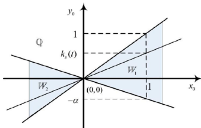
图 1 初值的指数吸引域
